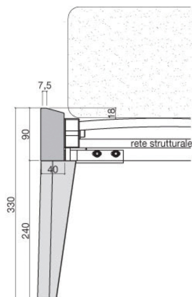
Sezione giroletto ALIANTE 2.0
