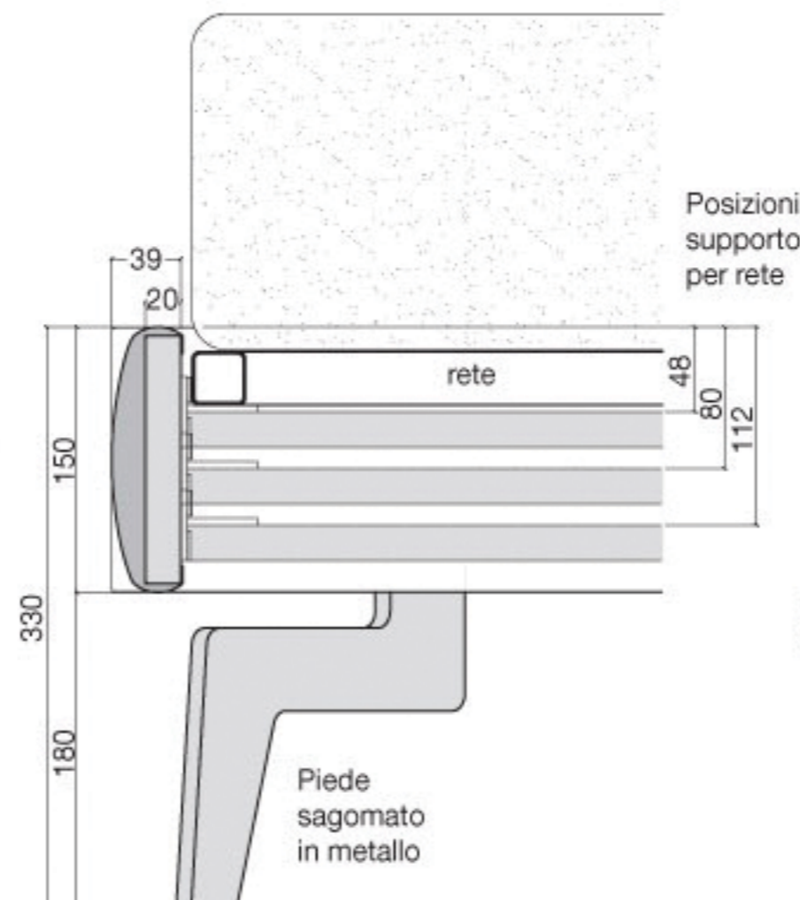
Sezione giroletto ALIANTE 3.0
